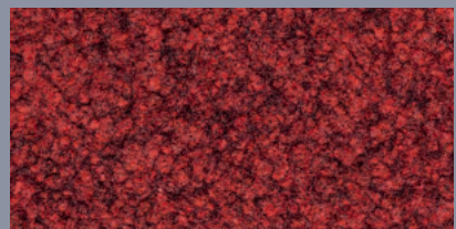
329 zirkon
