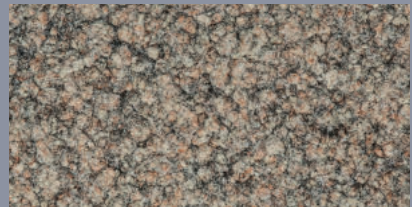
311 lehm
